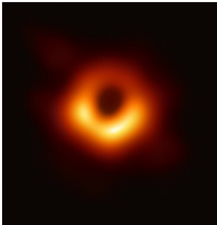
Image du trou noir supermassif M87* et de son disque d'accrétion. le 10 avril 2019
