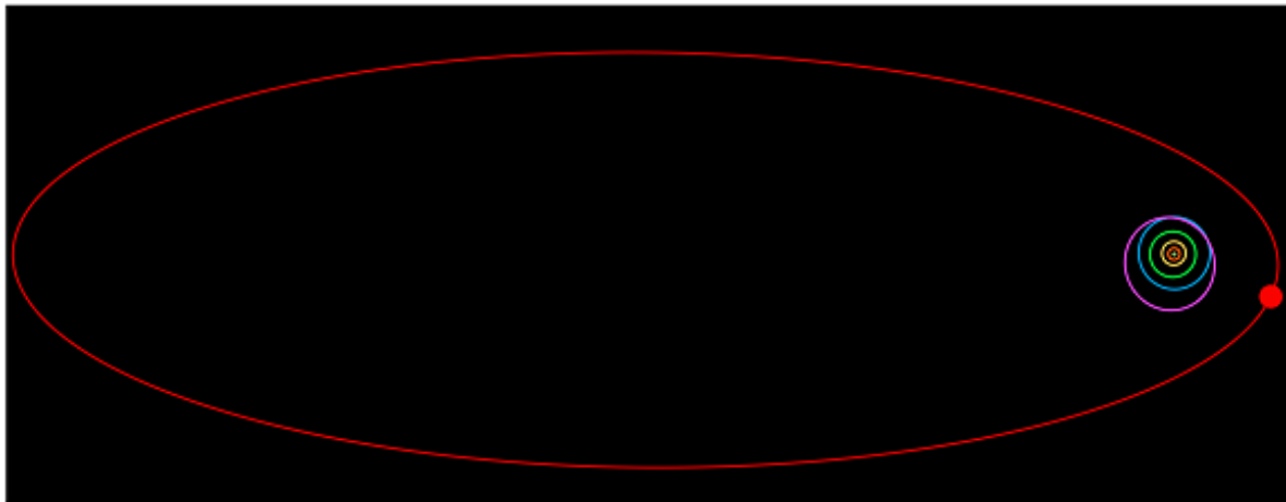
Orbite de Sedna
