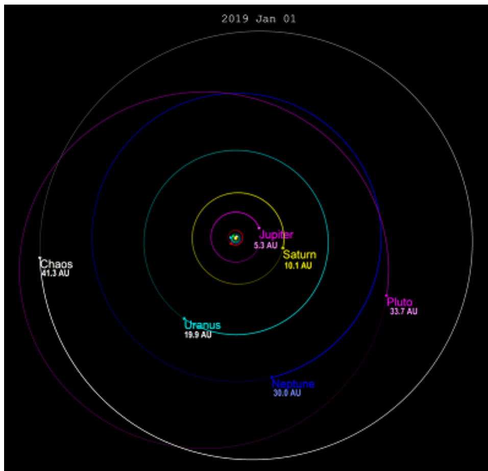
Orbite de (19521) Chaos par rapport à Pluton
