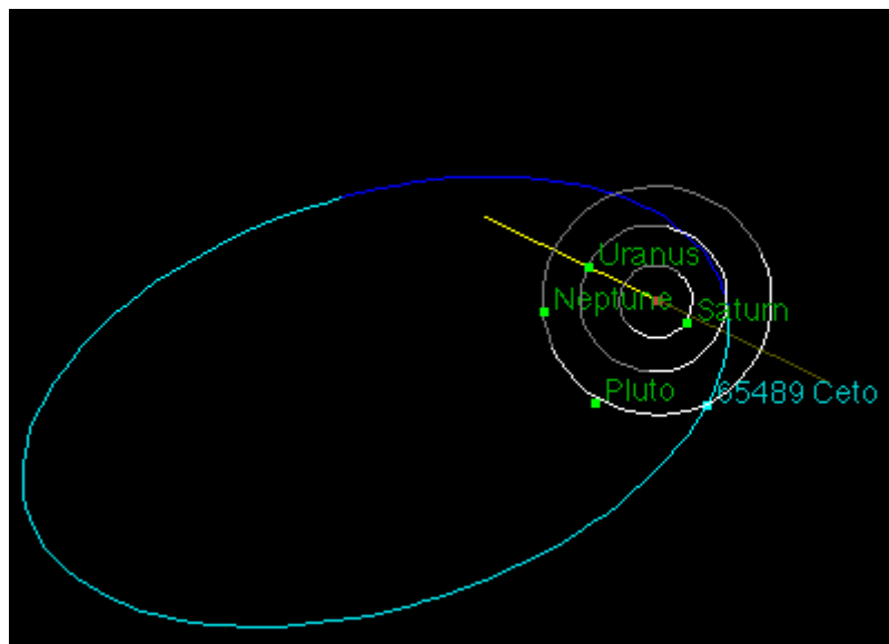
Orbite de (65489) Ceto
