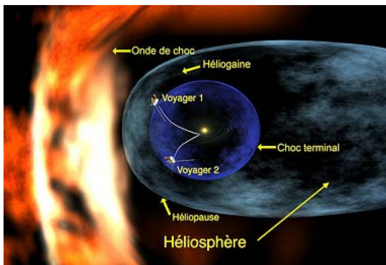
Schéma simplifié de l'héliosphère
