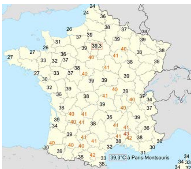
Températures maximales relevées en France le 12 août 2003, jour le plus chaud de l'année d'après Météo-France.
